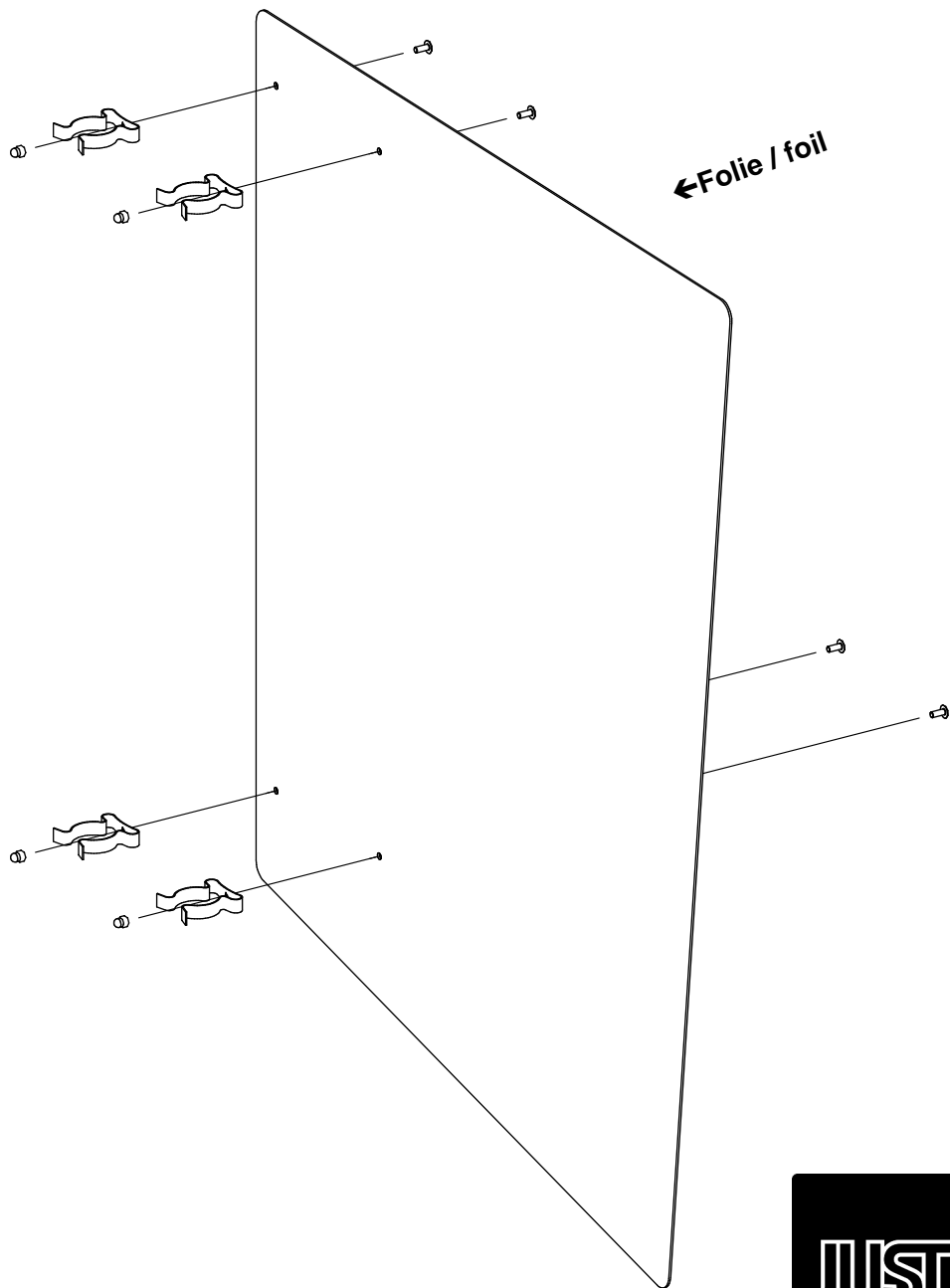
Seitenblende rechts Artikel-Nr. 4374 side wall right Item No. 4374
